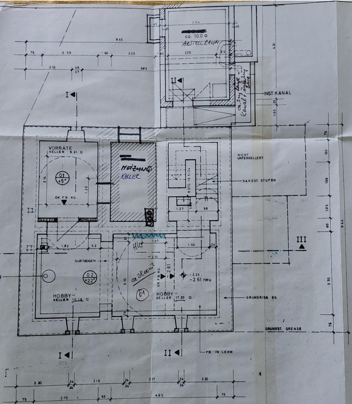
GRUNDRISS KELLERGEHOSS M. 1:50
